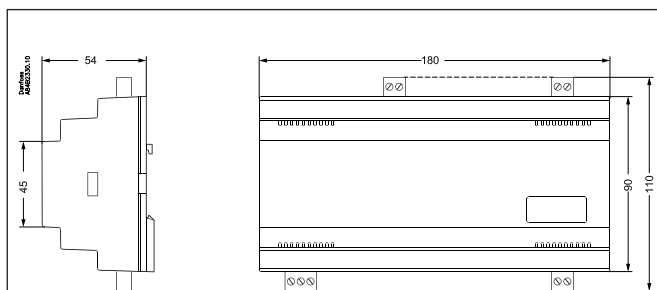
AK-PC 520
