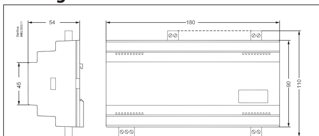
AK-PC 530
