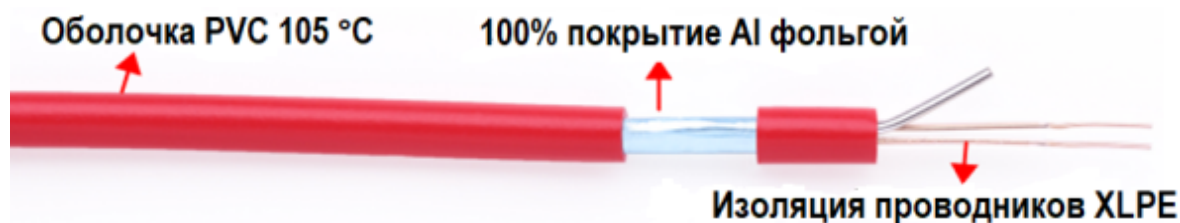
Рис. 2А. Оболочка, экран и изоляция проводников кабеля ДЕВИ Flex-10Т.
